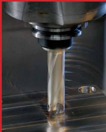
Werkzeuge und Wendeschneidplatten zum Bohren
