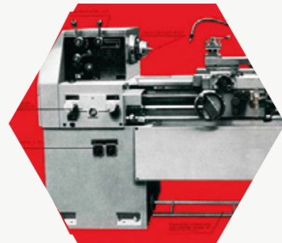
Erste Parallel-Dreimaschine
