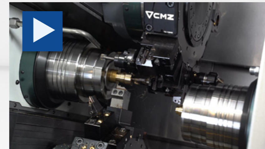
ÜBERLAGERTES GEWINDESCHNEIDEN
