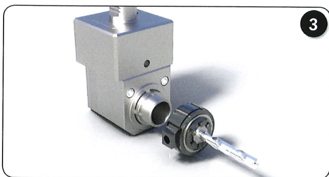
Montage reCool®, Dichtscheibe und IK-Werkzeug
