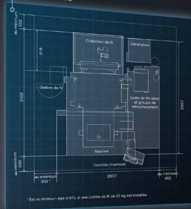
Plan de machine
